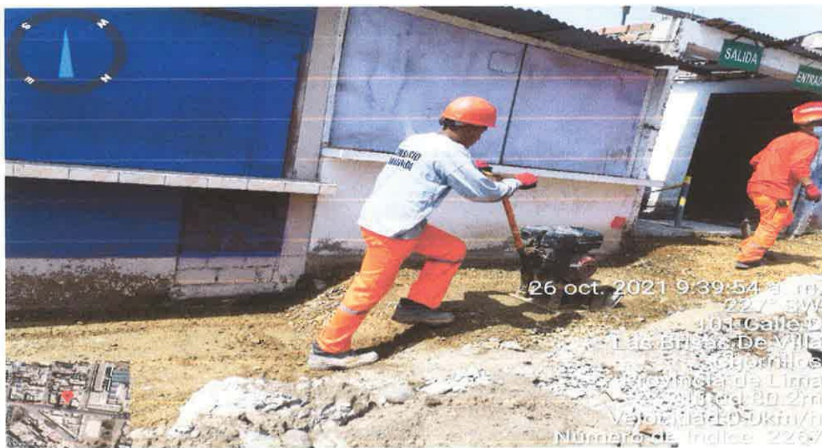
10. Conformación y compactación a nivel de sub rasante en veredas.
